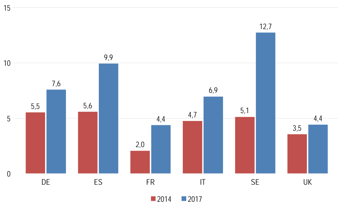
Abb. 2-4: Anteil der Unternehmen, die RFID (Radio Frequency Identification) Technologien einsetzen – Baugewerbe (in Prozent)
